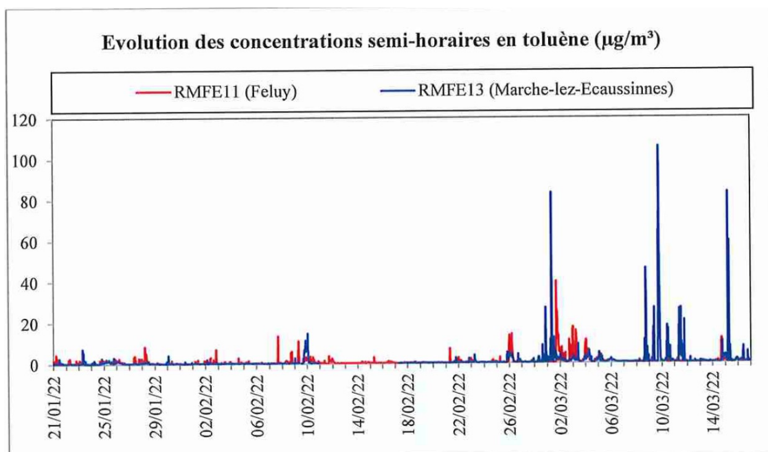
Figure 20 : Toluène – Evolution des concentrations semi-horaires (campagne Hiver 2022)
