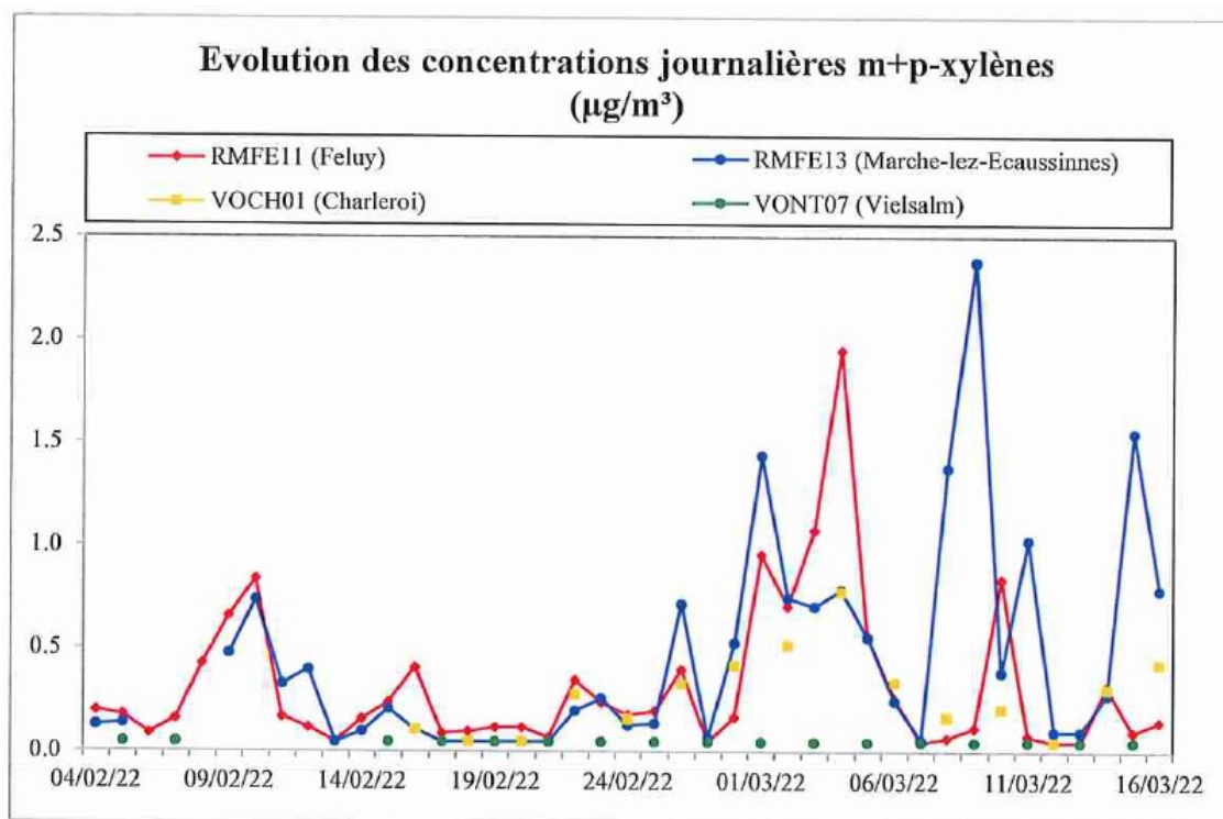
Figure 7.3.7 : m+p-xylènes – Evolution des concentrations journalières – Campagne « Hiver 2022 » (04/02/22 au 16/03/22)
