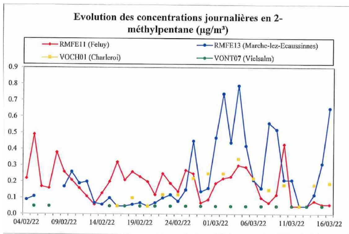
Figure 7.3.2 : 2-méthylpentane – Evolution des valeurs journalières – Campagne « Hiver 2022 » (04/02/22 au 16/03/22)
