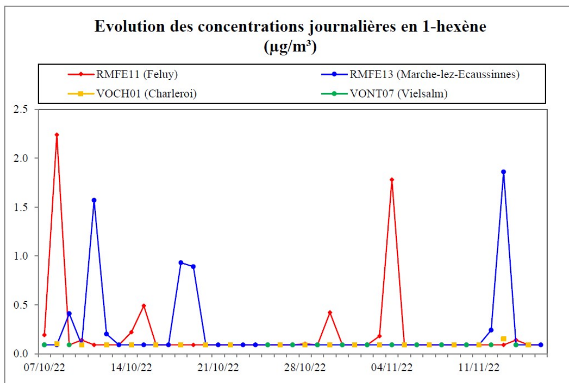
Figure 7.3.1 : 1-hexène – Evolution des concentrations journalières – Campagne « Automne 2022 » (07/10/22 au 16/11/22)
