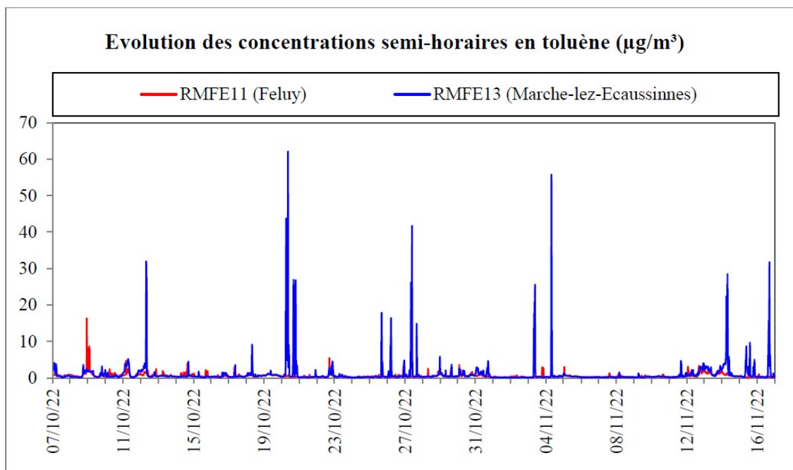
Figure 21 : Toluène – Evolution des concentrations semi-horaires (campagne Automne 2022)
