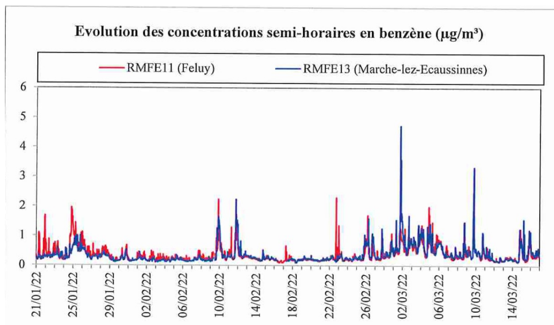
Figure 15 : Benzène – Evolution des concentrations semi-horaires (campagne Hiver 2022)
