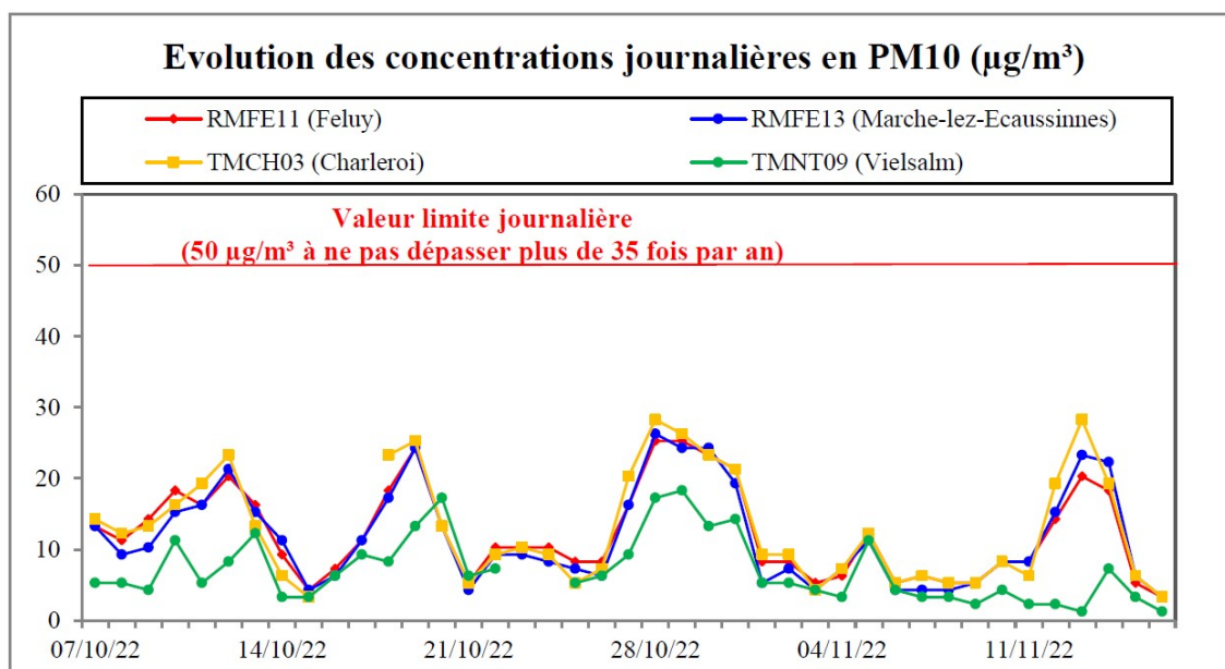
Figure 10 : Evolution des concentrations journalières de PM 10. (Campagne de mesure « automne 2022 ») - Source : ISSeP.
