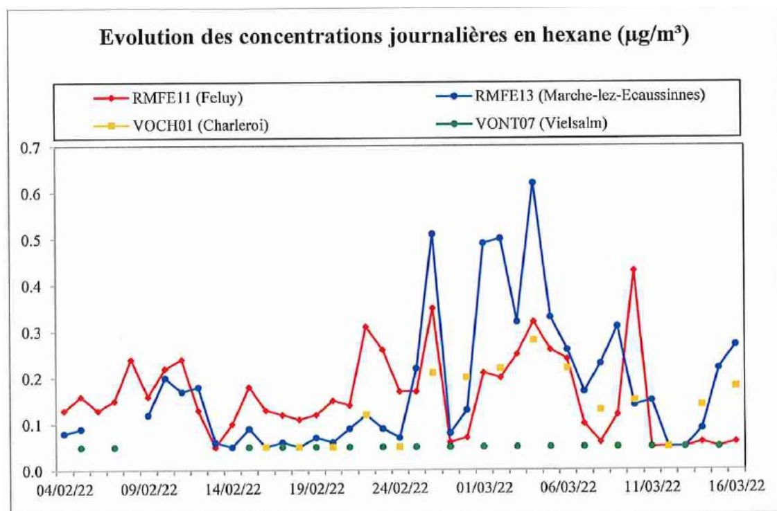
Figure 7.3.5 : hexane – Evolution des concentrations journalières – Campagne « Hiver 2022 » (04/02/22 au 16/03/22)
