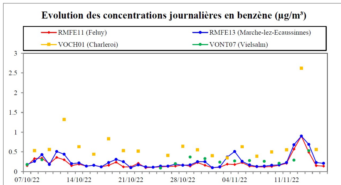
Figure 17 : Benzène – Evolution des concentrations journalières et comparaison avec des stations de référence (campagne automne 2022)
