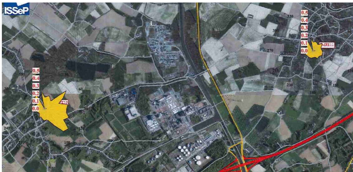
Figure 7.3.15 : heptane ( \mu\text{g}/\text{m}^3 ) – Roses de pollution – Campagne « Hiver 2022 » (04/02/22 au 16/03/22)
