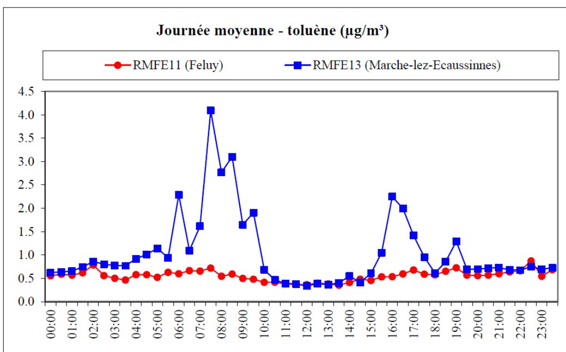
Figure 23 : Toluène – Evolution des concentrations lors de la journée moyenne (campagne Automne 2022)
