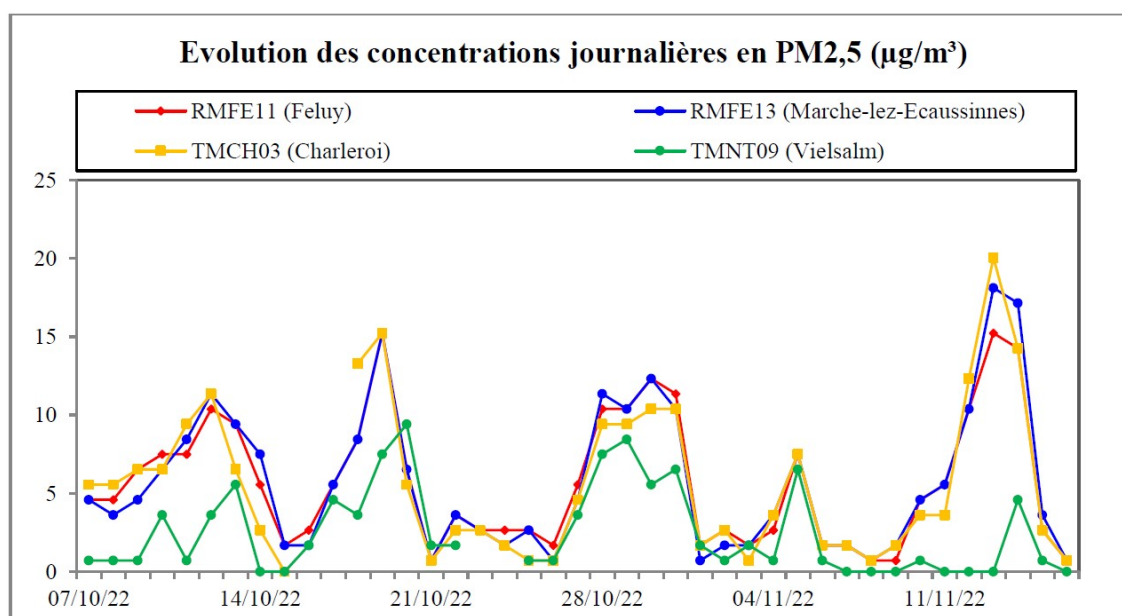
Figure 14 : Evolution des concentrations journalières de PM 2.5. (Automne 2022). Source : ISSeP.
