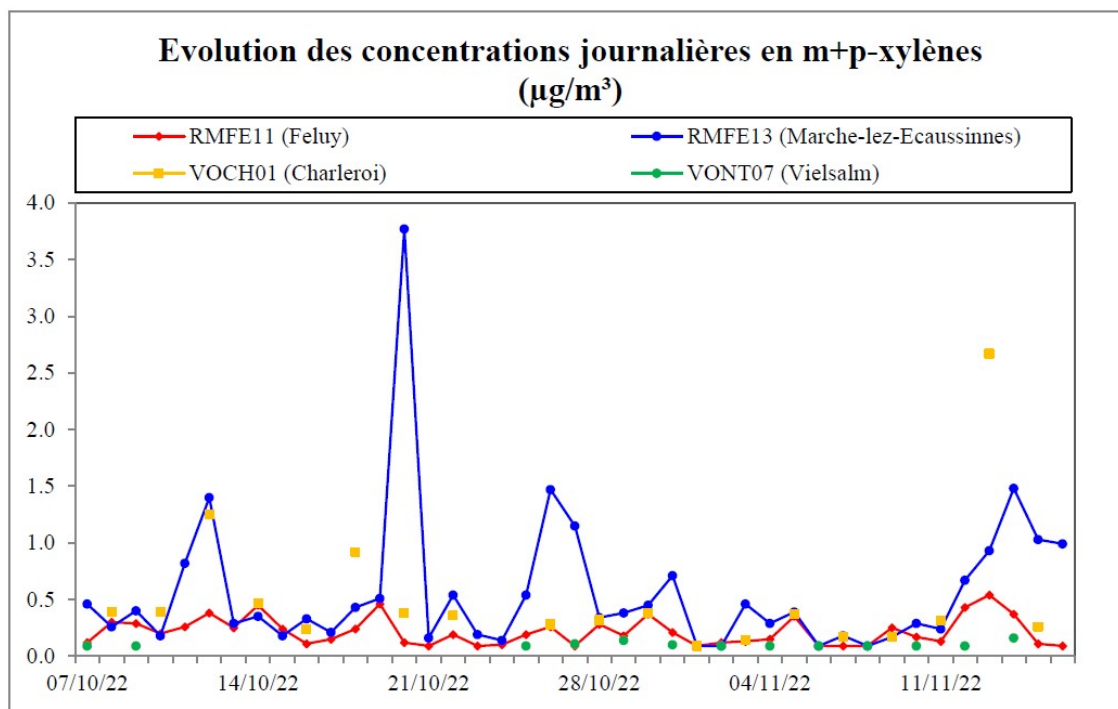
Figure 7.3.5 : m+p-xylènes – Evolution des concentrations journalières – Campagne « Automne 2022 » (07/10/22 au 16/11/22)
