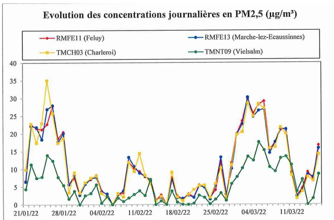
Figure 13 : Evolution des concentrations journalières de PM 2.5. (Hiver 2022). Source : ISSeP.
