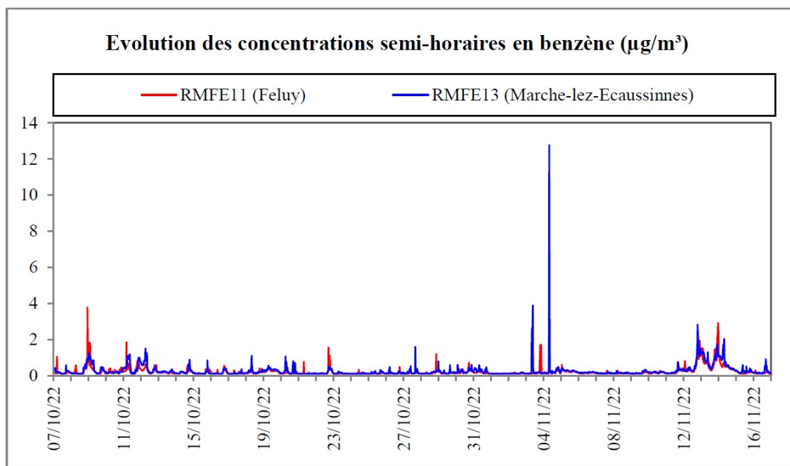
Figure 16 : Benzène – Evolution des concentrations semi-horaires (campagne automne 2022)
