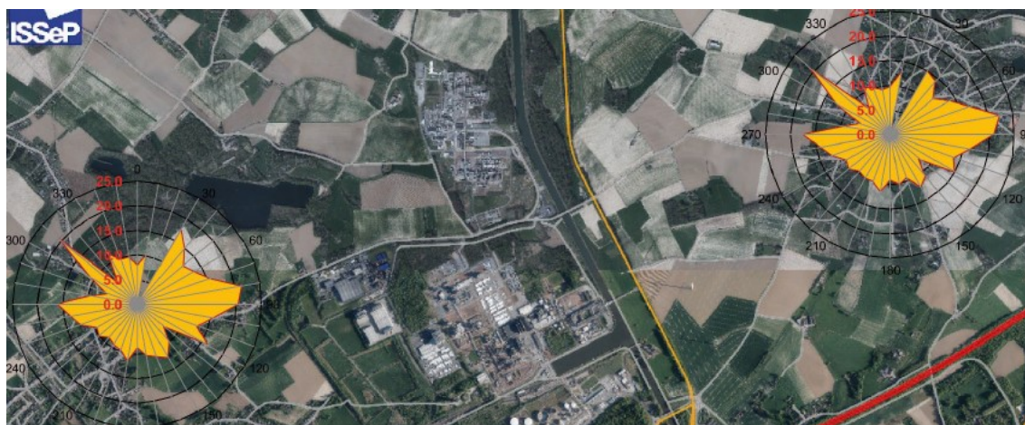
Figure 12 : Roses des pollutions pour les PM10 établies à l'automne 2022.
