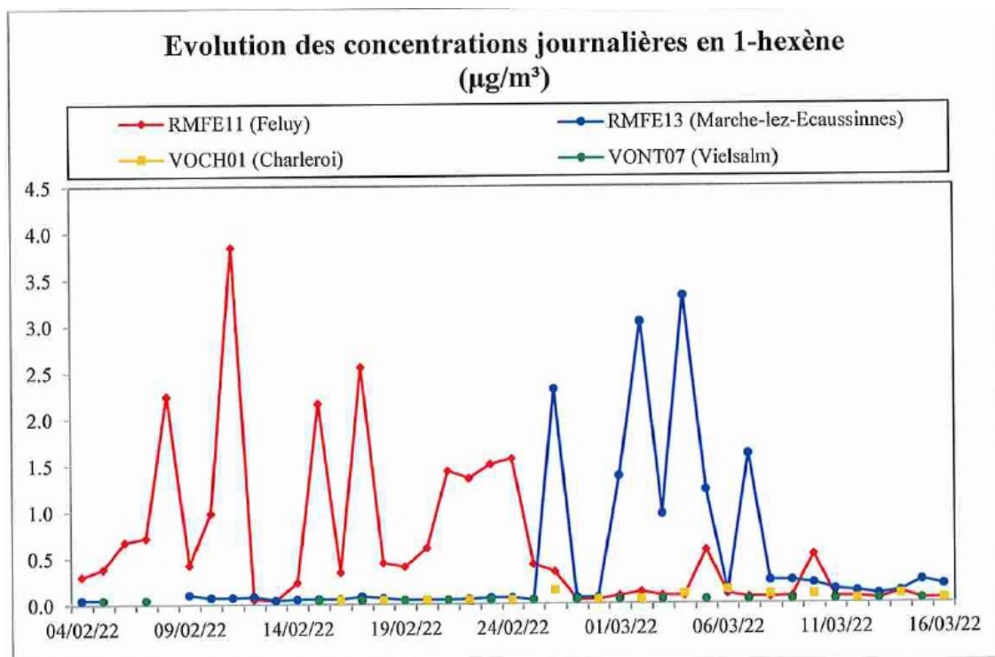
Figure 7.3.1 : 1-hexène – Evolution des concentrations journalières – Campagne « Hiver 2022 » (04/02/22 au 16/03/22)
