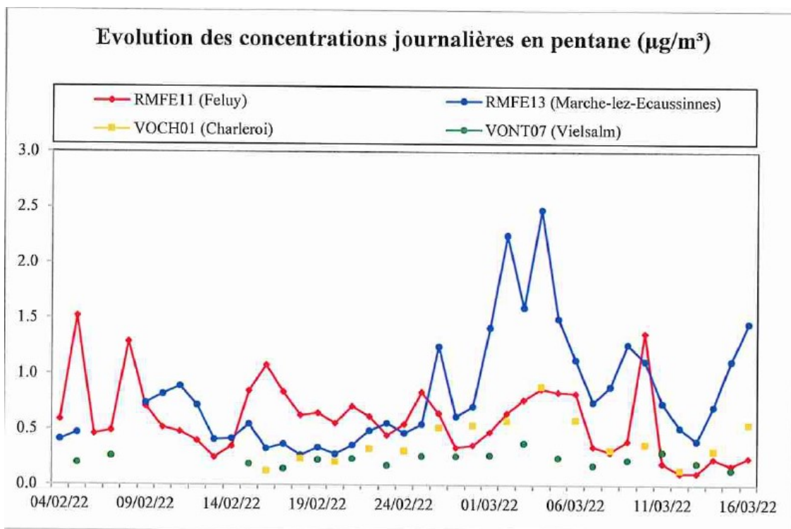
Figure 7.3.3 : pentane – Evolution des concentrations journalières – Campagne « Hiver 2022 » (04/02/22 au 16/03/22)
