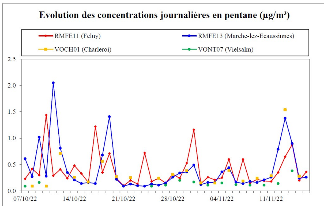
Figure 7.3.2 : pentane – Evolution des concentrations journalières – Campagne « Automne 2022 » (07/10/22 au 16/11/22)
