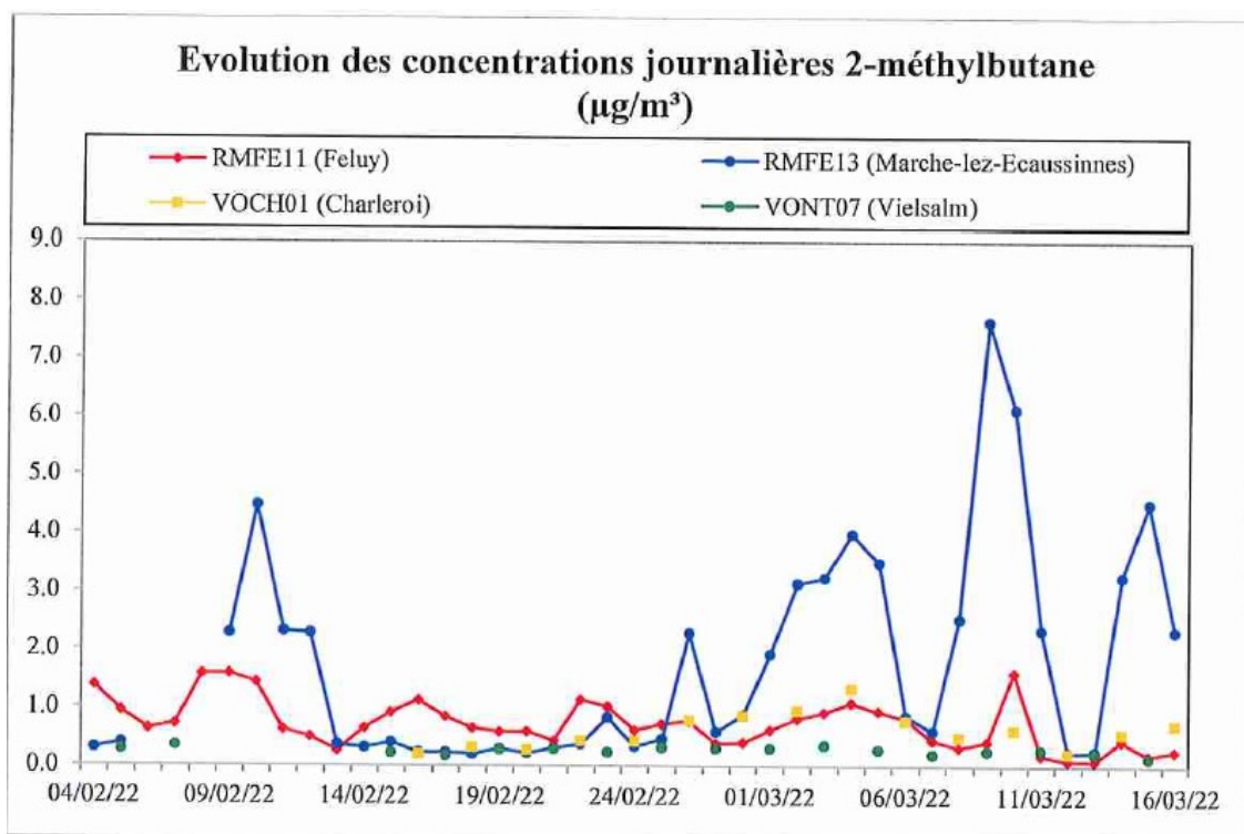
Figure 7.3.6 : 2-méthylbutane – Evolution des concentrations journalières – Campagne « Hiver 2022 » (04/02/22 au 16/03/22)
