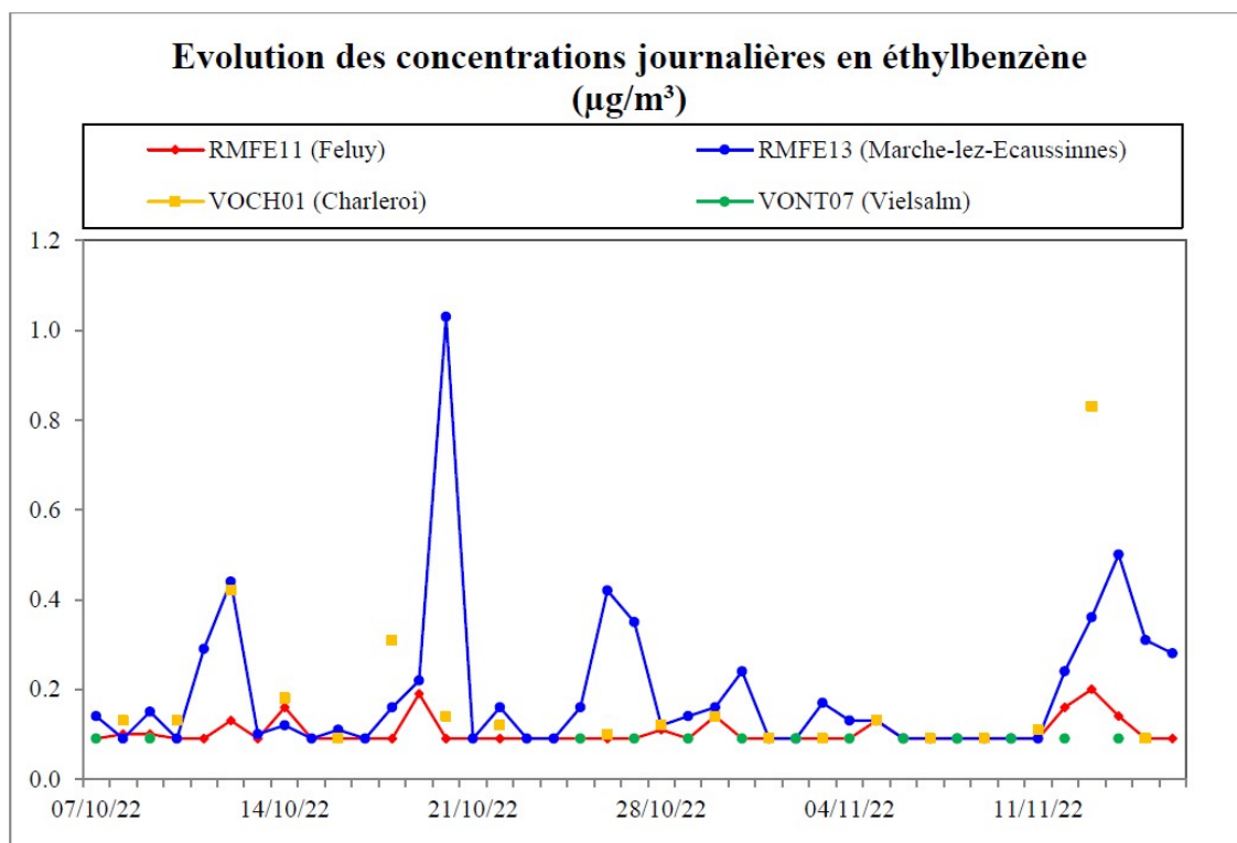
Figure 7.3.4 : éthylbenzène – Evolution des concentrations journalières – Campagne « Automne 2022 » (07/10/22 au 16/11/22)
