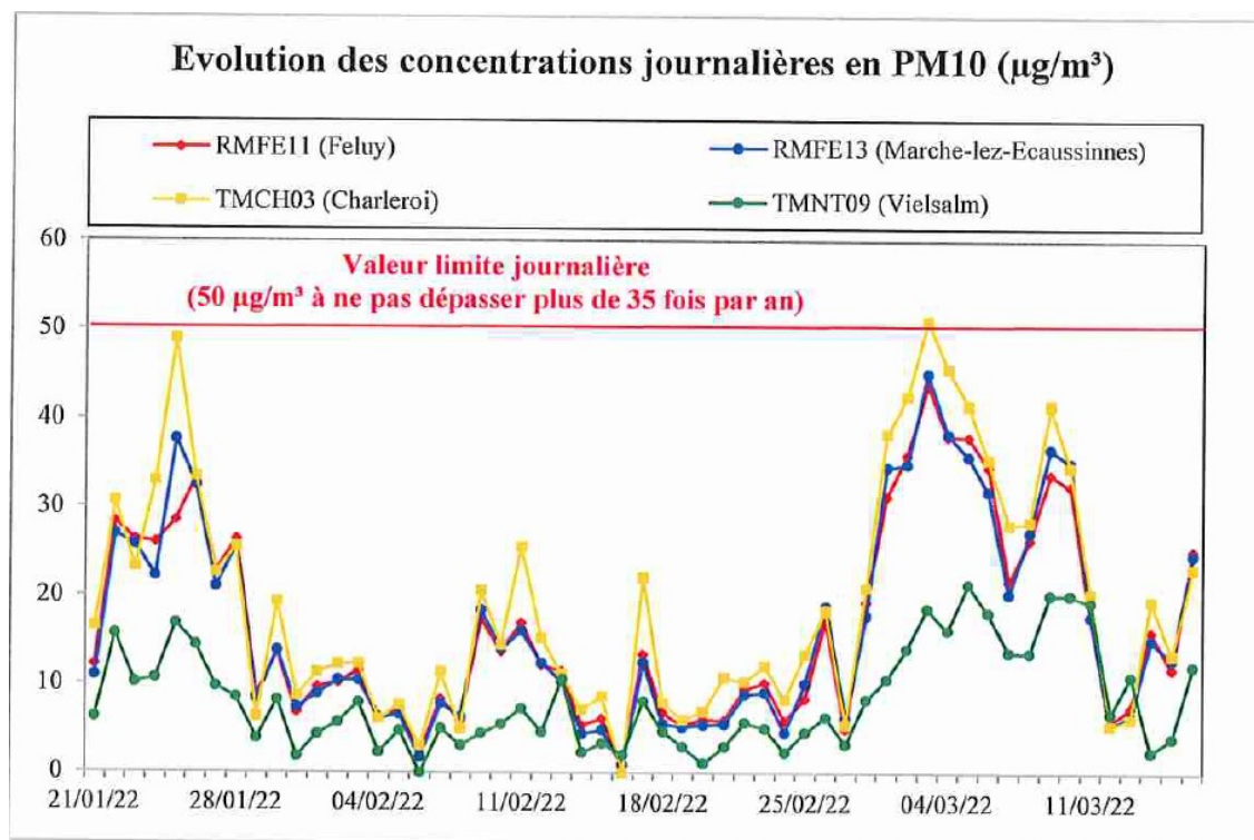
Figure 9 : Evolution des concentrations journalières de PM 10 (hiver 2022).
