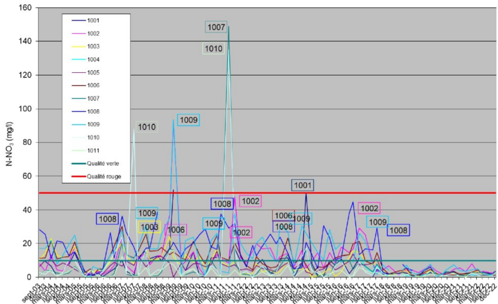
Figure 36 : Historique des concentrations de nitrate s depuis septembre 2003 jusqu'à 2022.
