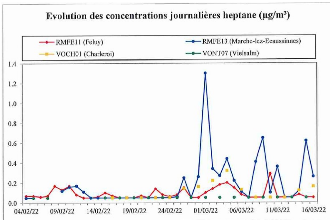
Figure 7.3.8 : heptane – Evolution des concentrations journalières – Campagne « Hiver 2022 » (04/02/22 au 16/03/22)
