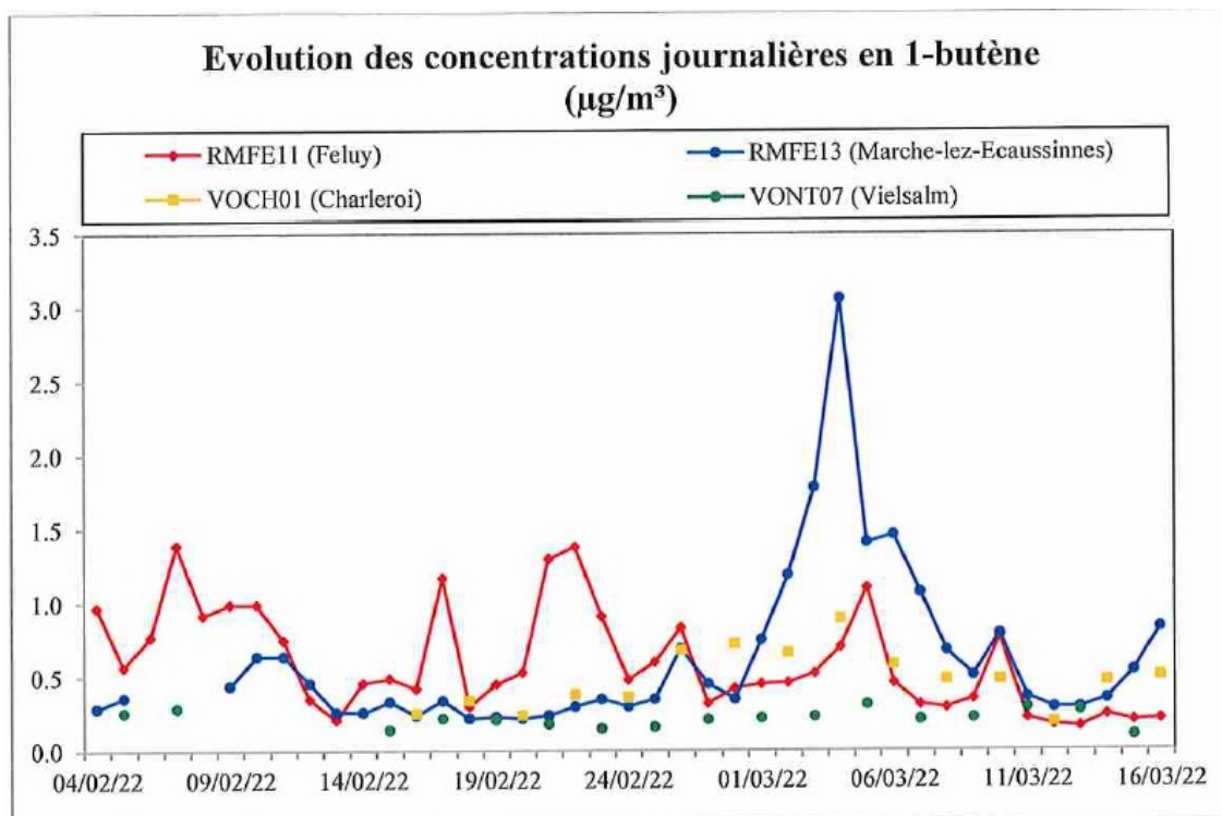
Figure 7.3.4 : 1-butène – Evolution des concentrations journalières – Campagne « Hiver 2022 » (04/02/22 au 16/03/22)
