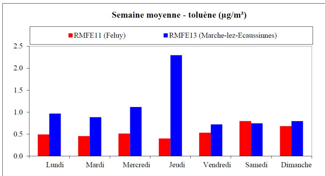
Figure 24 : Toluène – Evolution des concentrations lors de la semaine moyenne (campagne Automne 2022)
