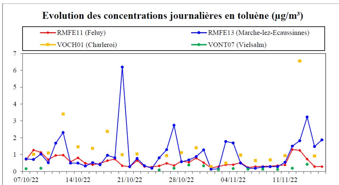
Figure 22 : Toluène – Evolution des concentrations journalières (campagne Automne 2022)
