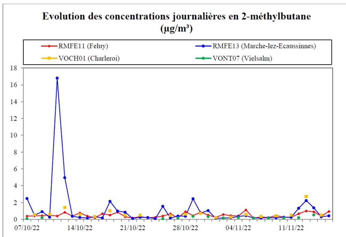
Figure 7.3.3 : 2-méthylbutane – Evolution des concentrations journalières – Campagne « Automne 2022 » (07/10/22 au 16/11/22)
