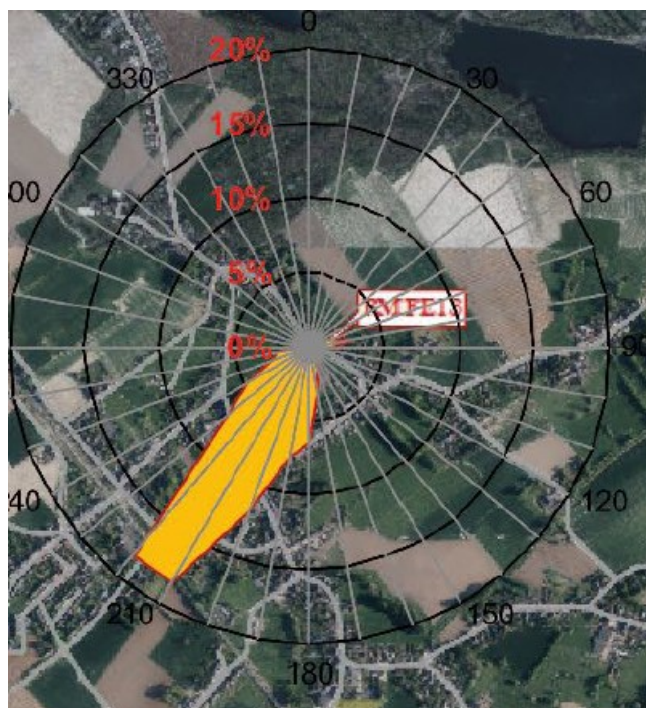
Figure 8 : Rose des vents à Marche-lez-Ecaussinnes lors de la deuxième campagne de mesure 2022.
