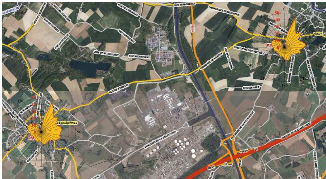
Figure 11 : Roses des pollutions pour les PM10 établies au printemps 2015.
