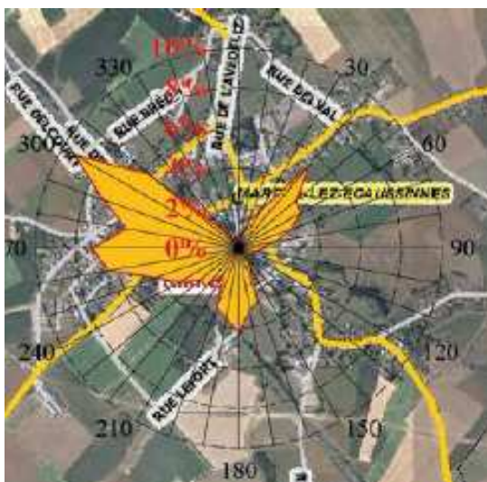
Figure 7 : Rose des vents à Marche-lez-Ecaussinnes lors de la campagne de mesure 2015 du 18/03/2015 au 26/05/2015).
