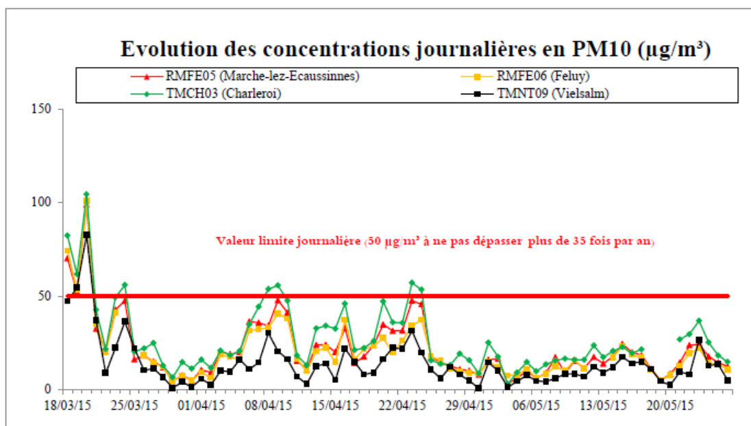
Figure 9 : Evolution des concentrations journalières de PM 10 . (18/03/2015 au 26/05/2015)
