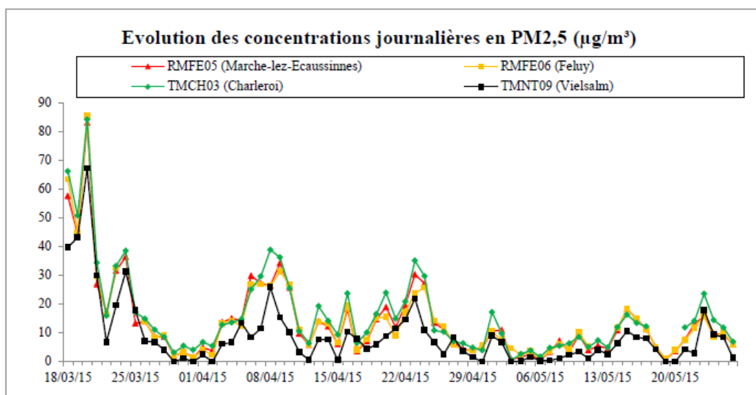
Figure 13 : Evolution des concentrations journalières de PM 2.5. (18/03/2015 au 26/05/2015)
