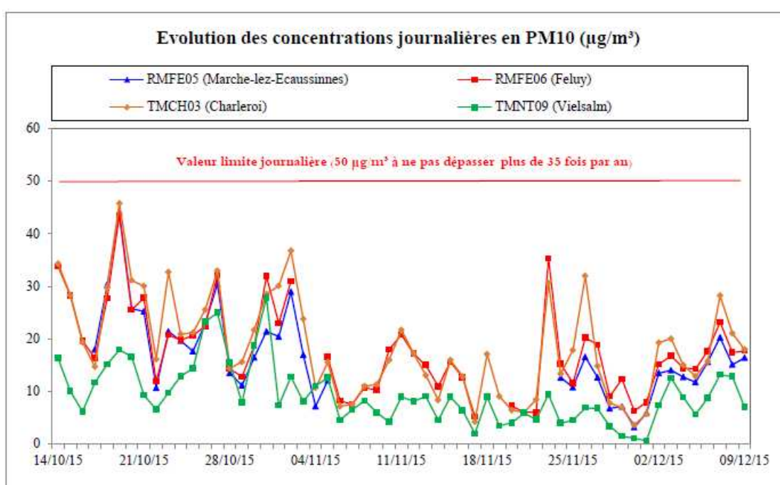
Figure 10 : Evolution des concentrations journalières de PM 10. (14/10/2015 au 09/12/2015)
