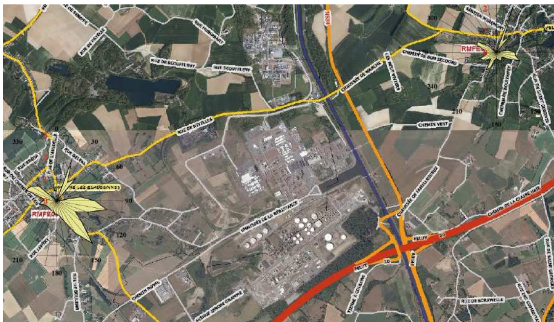
Figure 18 : Toluène ( \mu\text{g}/\text{m}^3 ) – Roses de pollution (14/10/2015 au 09/12/2015)
