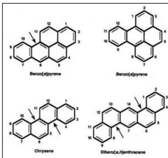
Figure 15 : Représentation de quelques Hydrocarbures Aromatiques Polycycliques (HAP).
